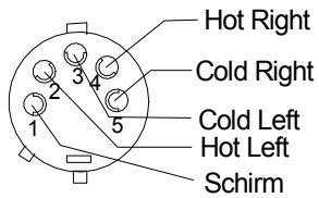
Rückansicht ( Normal ) XLR - Male 5 Pol
