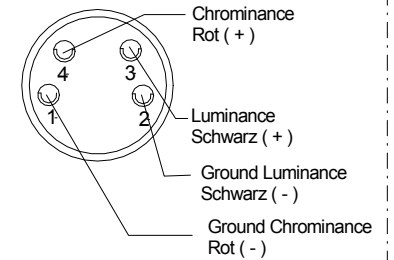
Rückansicht Y/C - S4P
