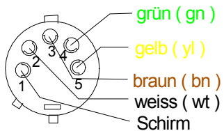
DMX-Belegung Rückansicht XLR - Male 5 Pol
