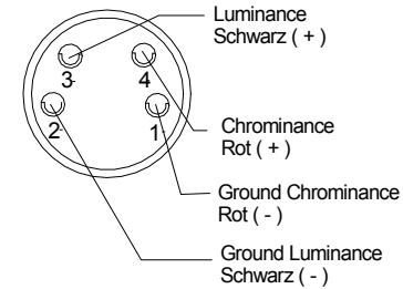
Rückansicht Y/C - S4J
