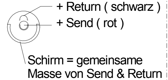
Rückansicht Plug Stereo für Insertverbindungen
