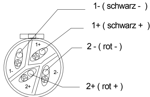
NL4FX mit ZNK 4/11
