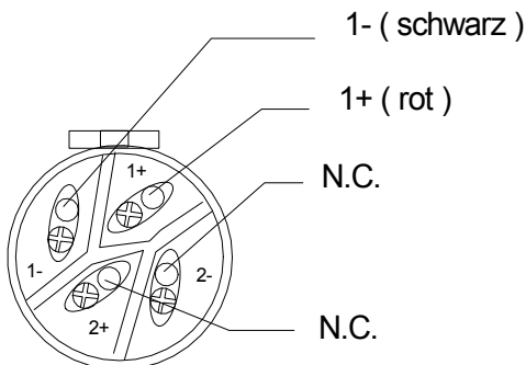
NL4FX mit ZNK 2/9
